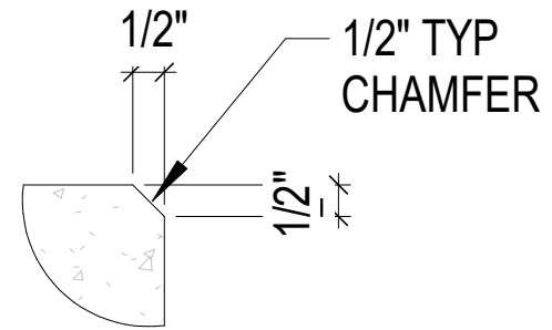
TYP PANEL EDGE
